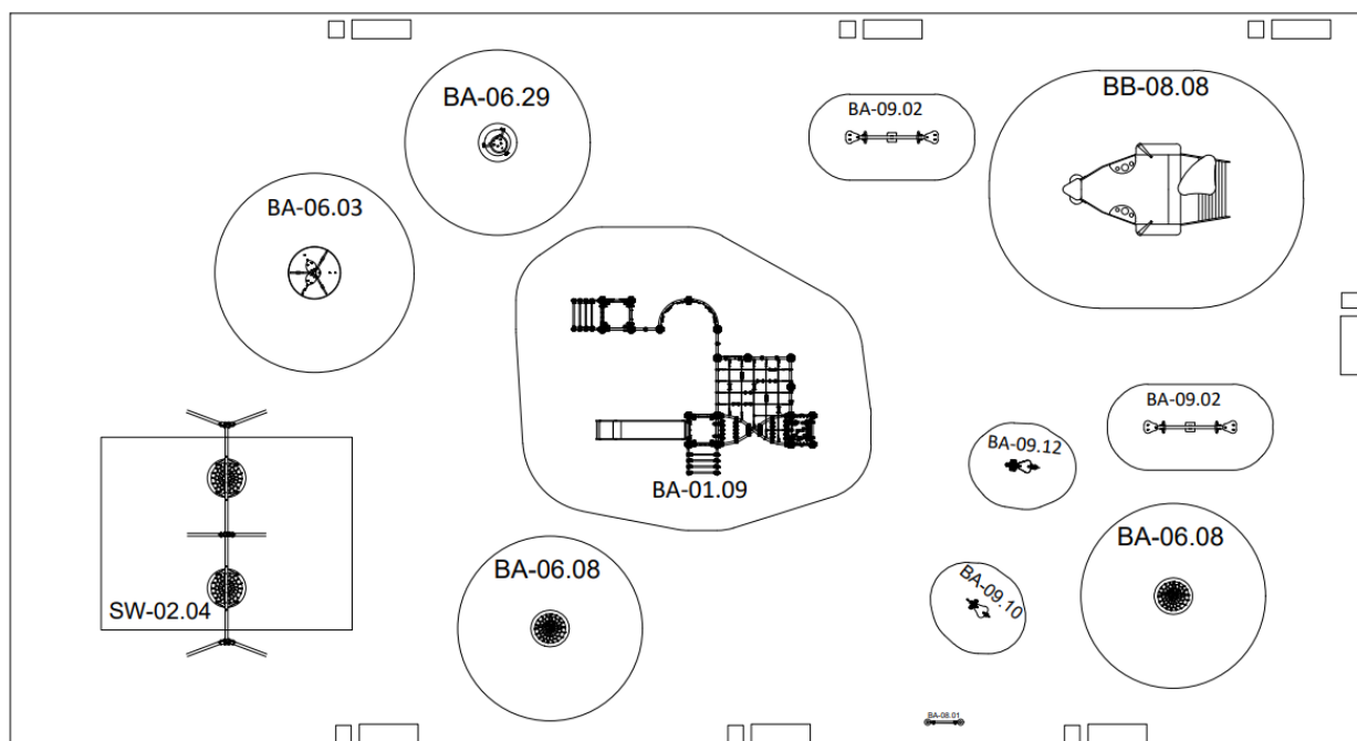
10.5.3. Спецификация элементов оборудования для установки.
