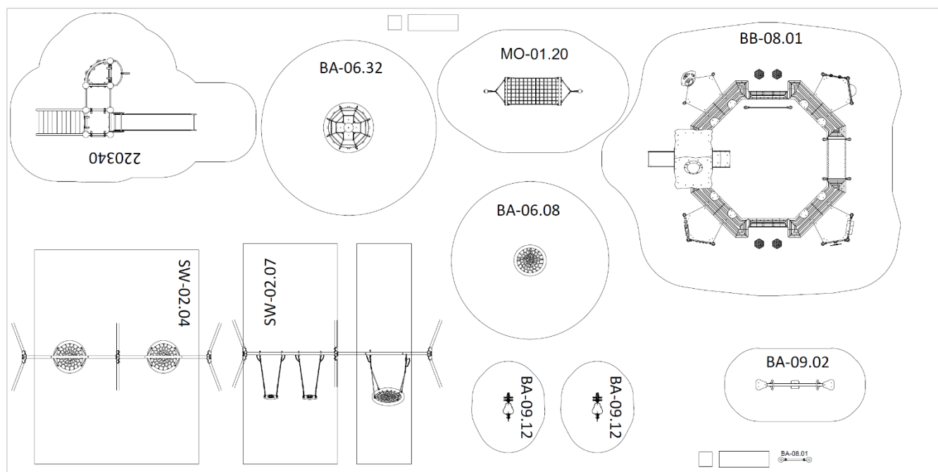
10.1.3. Спецификация элементов оборудования для установки.
